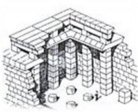
شكل رقم (٣) يوضح الفتحات العلوية الرأسية - سقف معبد الكرنك
